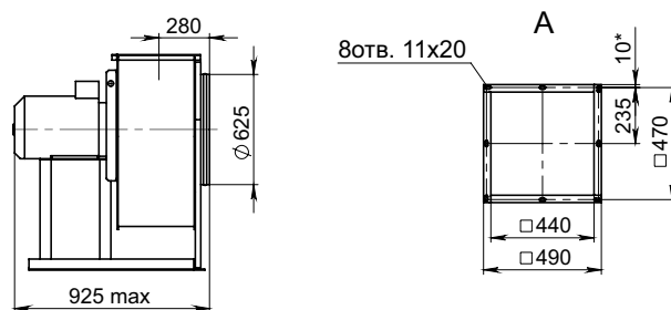
Вариант изготовления с входным ниппелем
