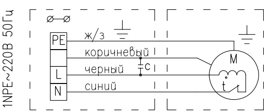
Схема Б. Подключение к сети 220 В 50 Гц
